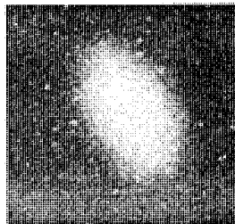
کهکشان بیضوی NGC147
