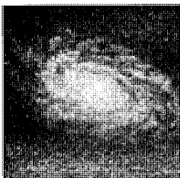
کپکشان مارپیج NGC4414
