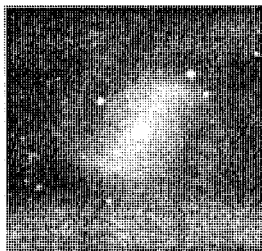
کهکشان میله مارپیج NGC4314
